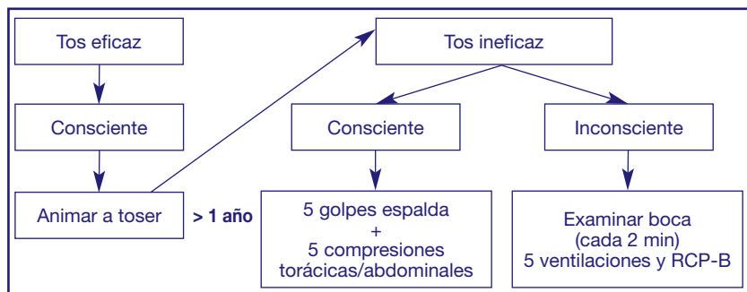
Figura 161.7. Algoritmo OVACE.
